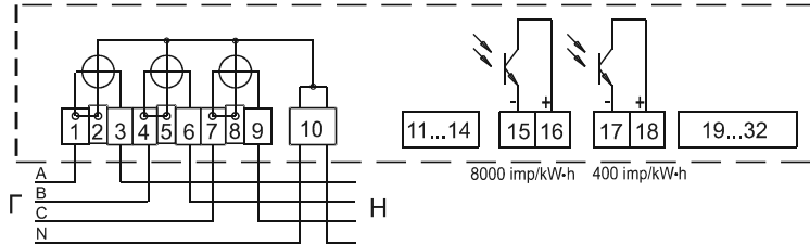
Рисунок 1 - Схема підключення лічильника
